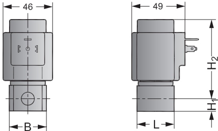
线圈类型 BQ，BB
