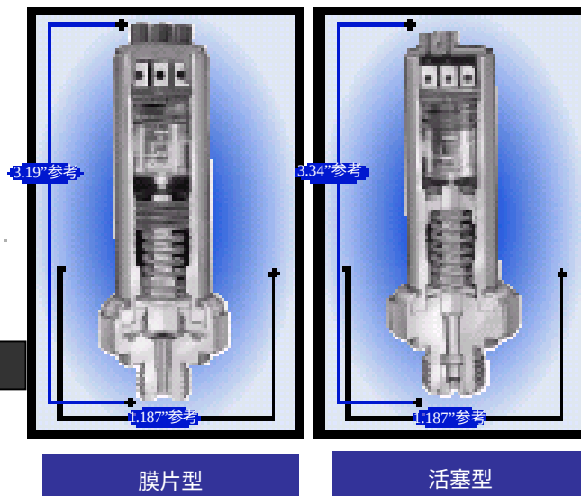
膜片型
